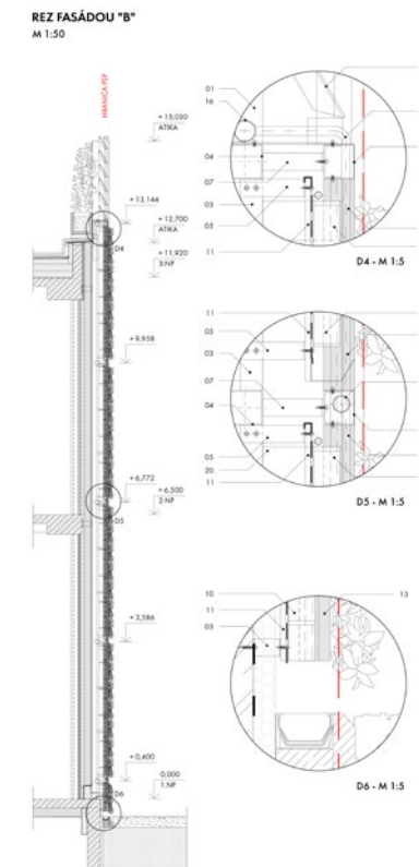
Řez fasádou
