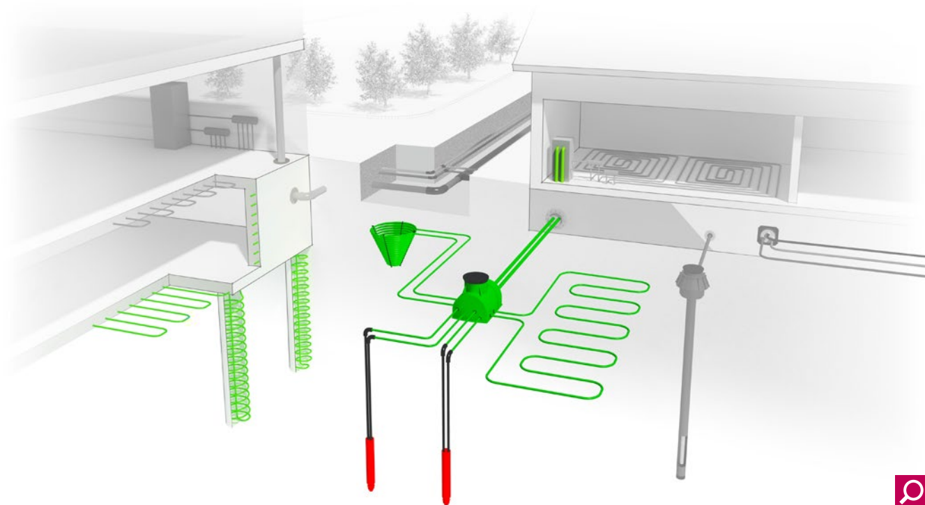
Systémy mělké geotermie ve schématu
